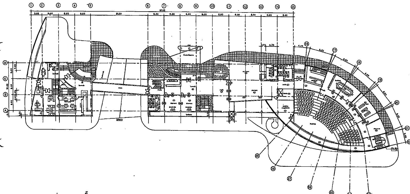
แบบแปลนพื้นชั้น 1 อาคาร A สำนักงานศุลกากรและศูนย์ราชการ 1:400 1ST FLOOR PLAN bld.-A custom and OneStopService government center 1:400
