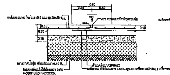
แบบขยาย ข. รอยต่อเพื่อการหดตัว (CONTRACTION JOINT) 1:10
