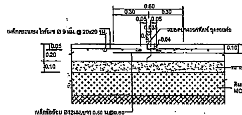
แบบขยาย ก. รอยต่อตามยาว (LONGITUDINAL JOINT) 1:10
