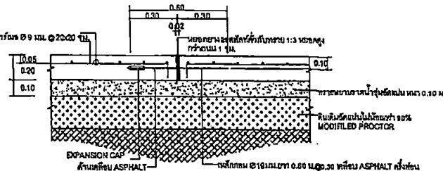
แบบขยาย ค. รอยต่อเพื่อการขยายตัว (EXPANSION JOINT) 1:10
